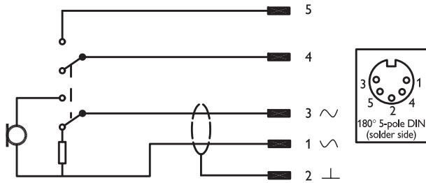
电路图
