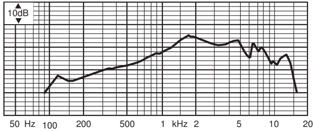
频率响应
